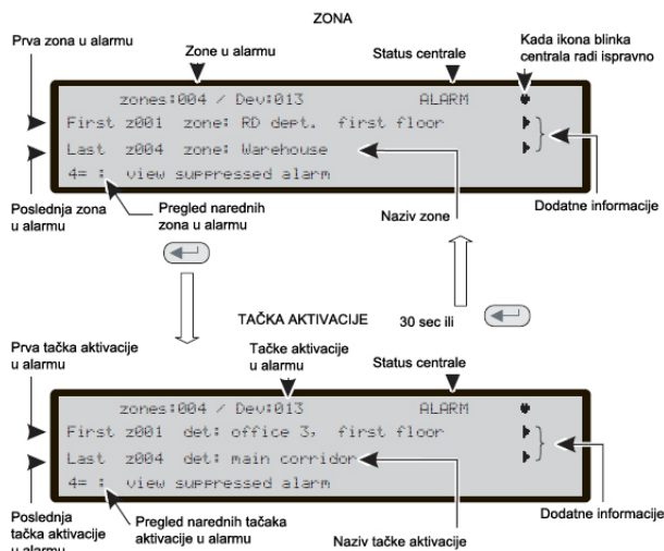
Slika 12 Alarm - prikaz na LCD displeju
